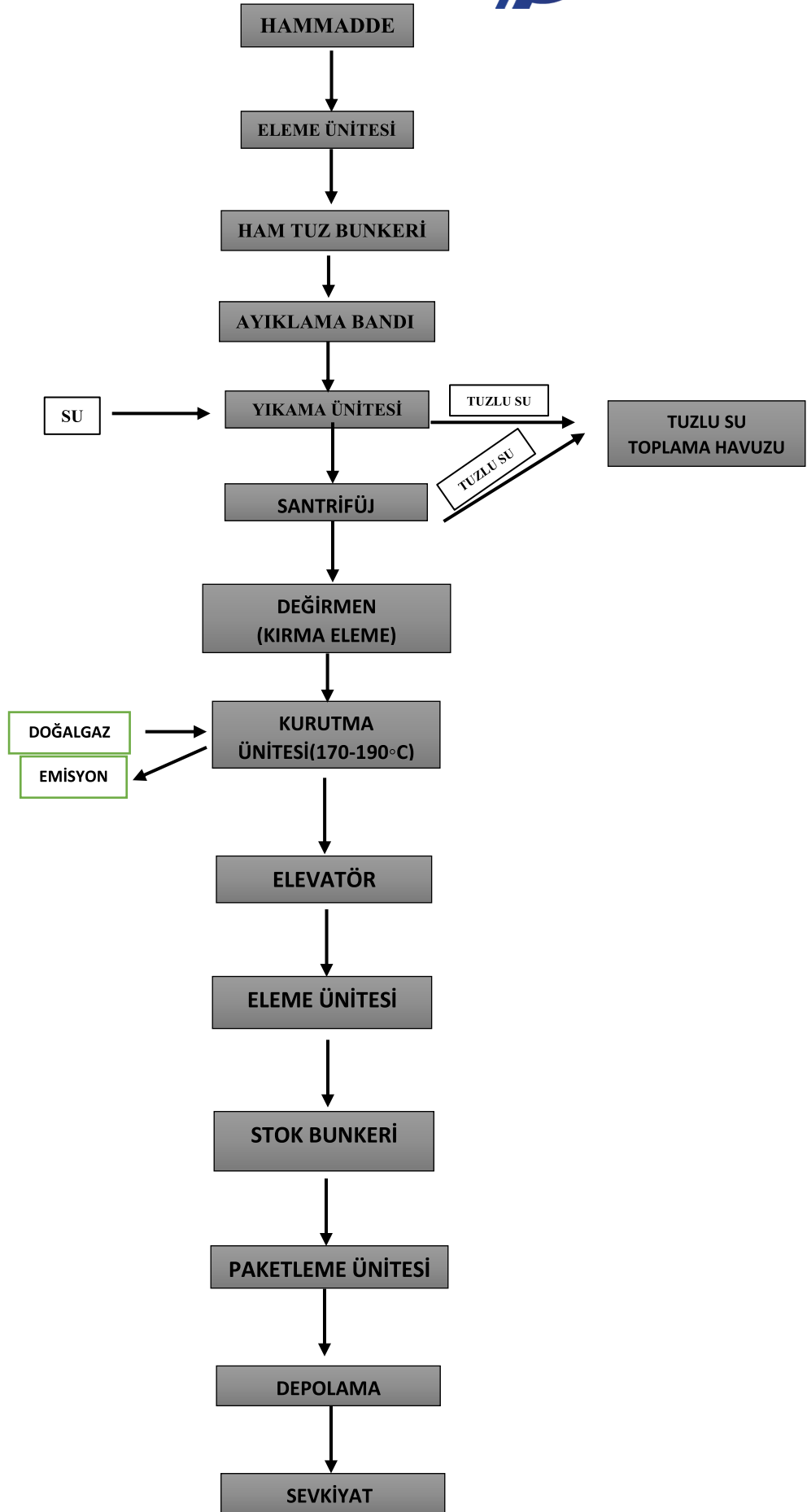
Şekil 1. TUZ İş Akım Şeması
